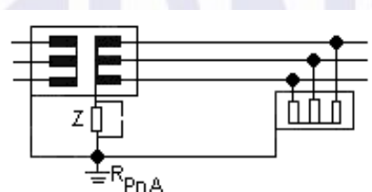
Figura 5 — Esquema ITS
