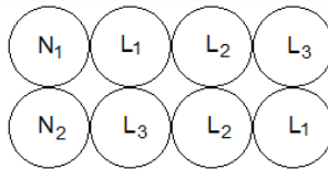
Figura 10 – Seis cabos unipolares, um acima do outro
